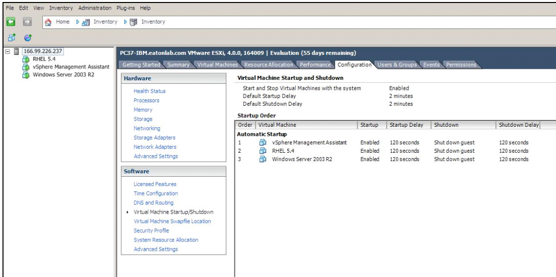
圖 82。vCenter 頁面
