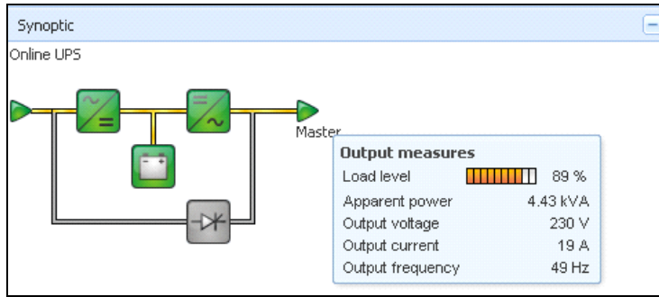
圖 56。概要面板
