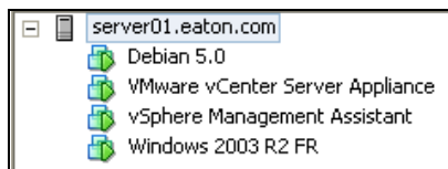
圖 87。階層選擇
